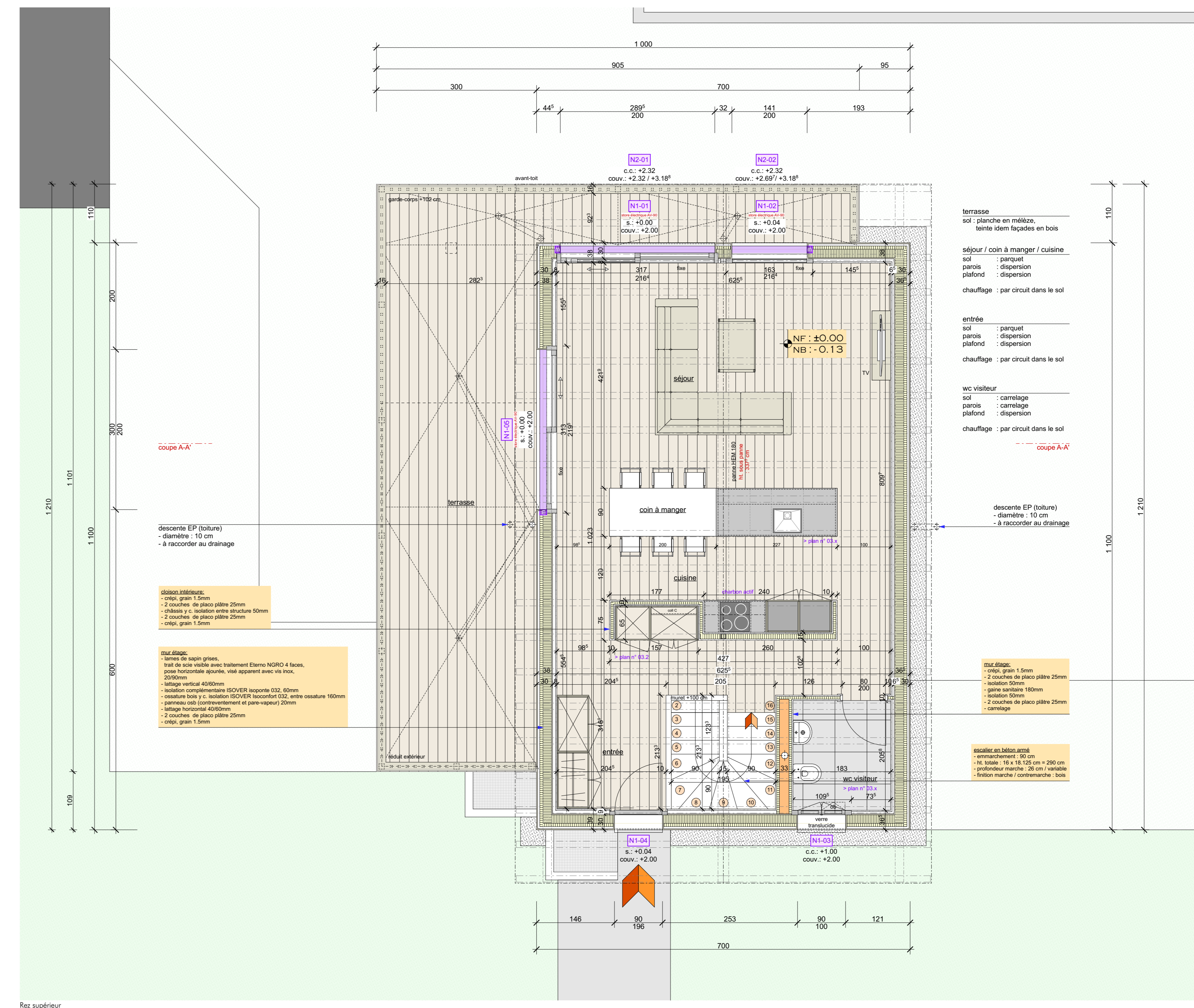
Rez supérieur
