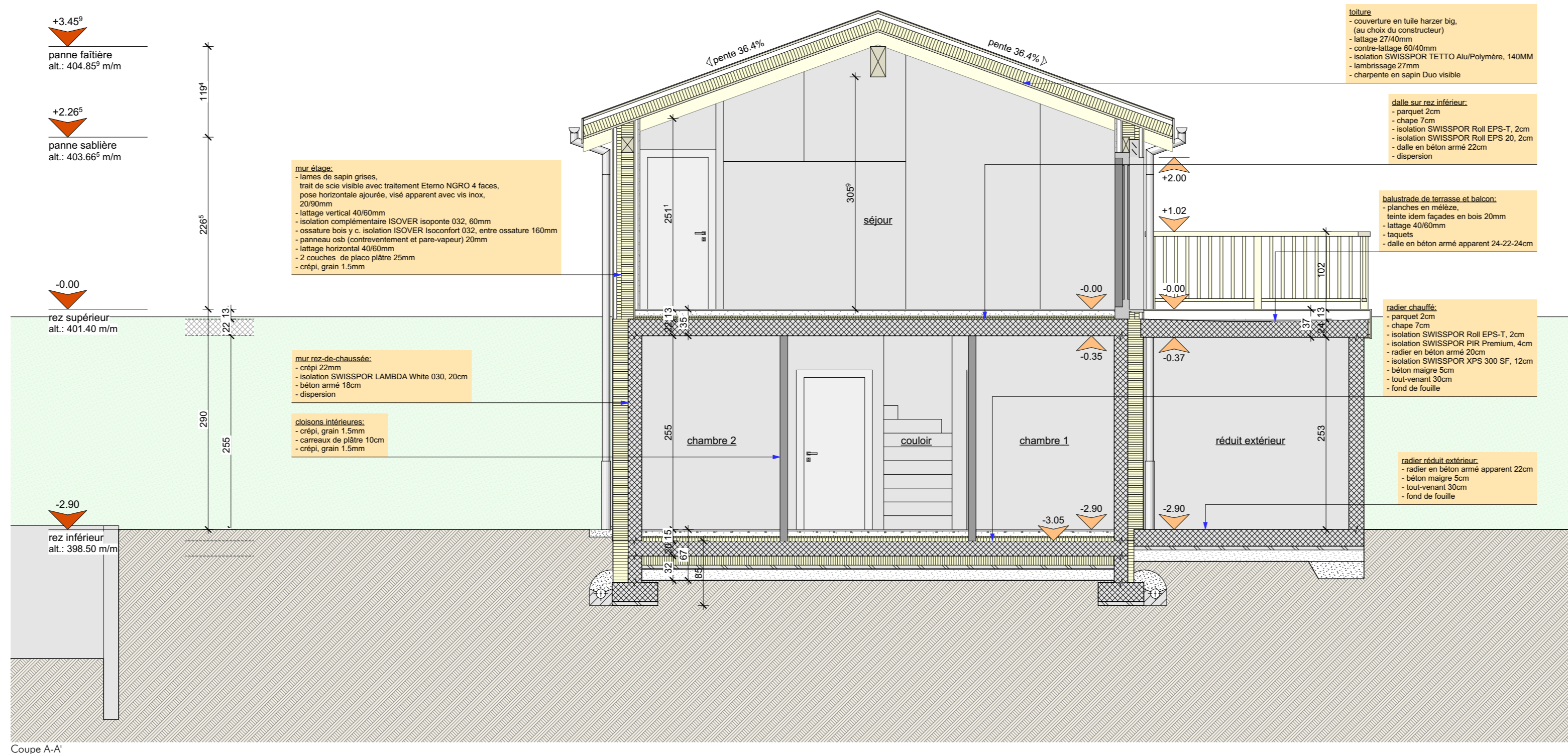
Coupe A-A
