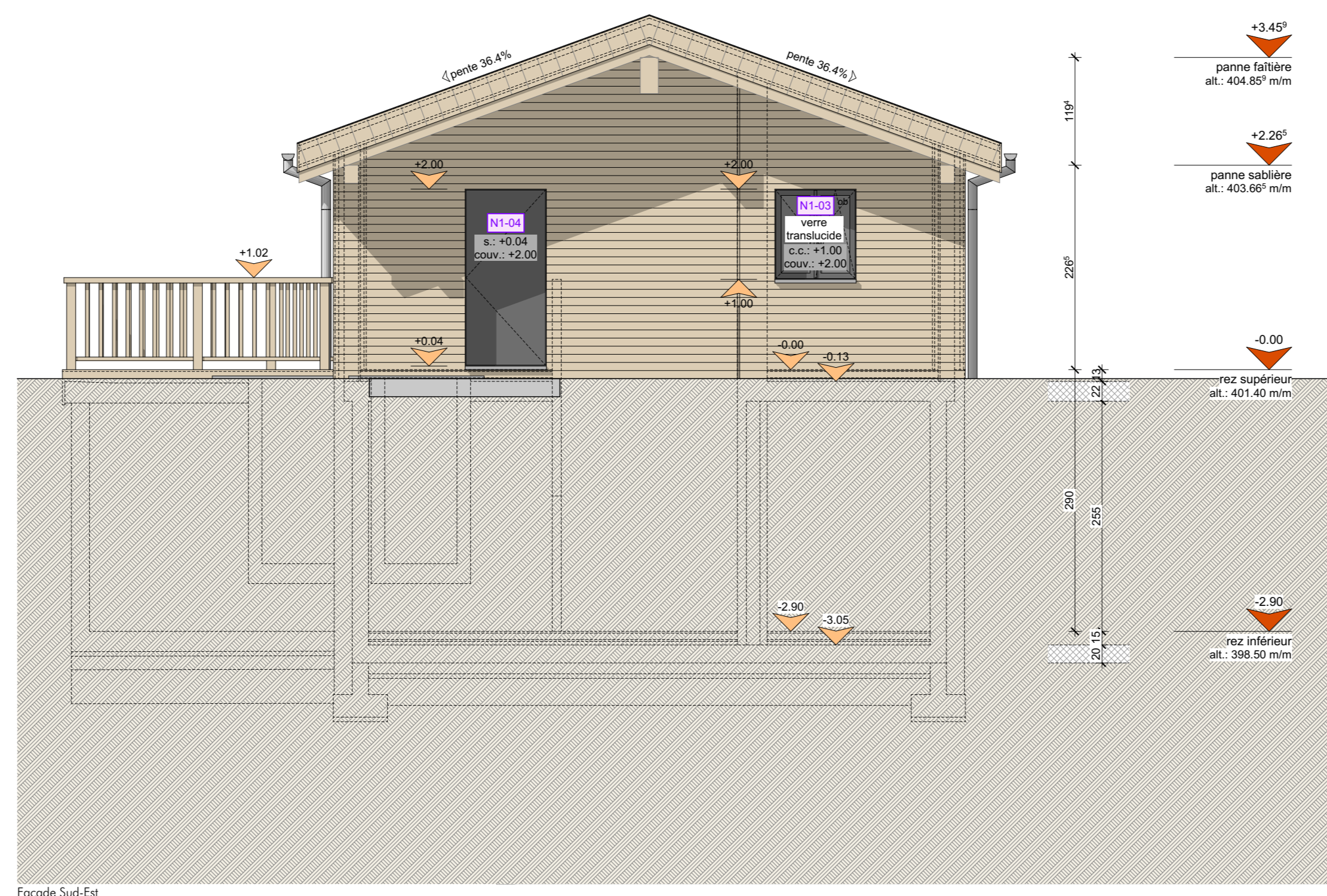
Façade Sud-Est
